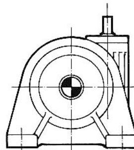
SPV mit freier Antriebswelle with free input shaft avec arbre d'entrée libre
